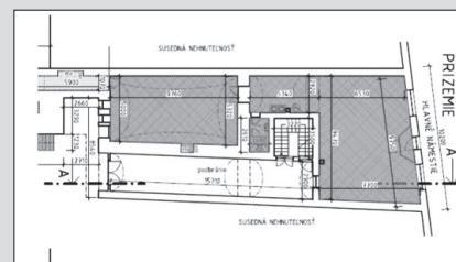
Pôdorys.
